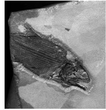
Caturus tarraconensis
