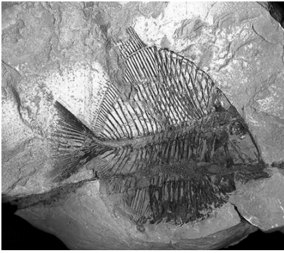
Ocloedus subdiscus
